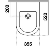
BIDET SOSPESO
