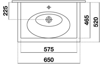
LAVABO A CONSOLLE 65
