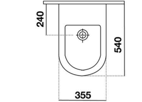
BIDET A PAVIMENTO
