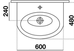
LAVABO 60
